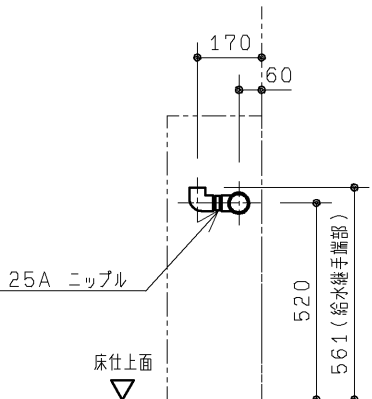
Q 視図
