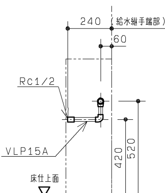
R 視図
