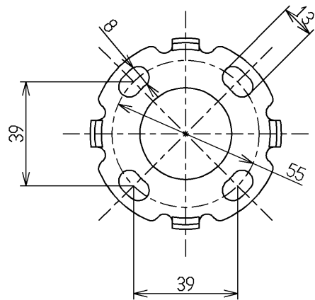
取付座詳細(1:2)
