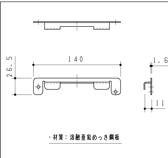
ソケット押え板
