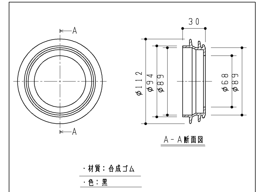
排水パッキン
