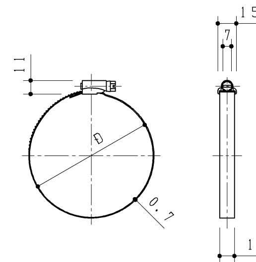
ホースバンド(2ヶ)
