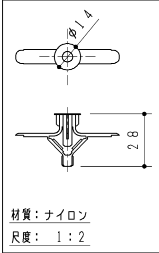
ボードアンカー 6ヶ
