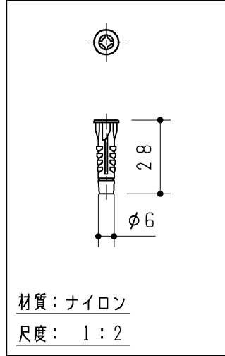
ボードアンカー 7ヶ
