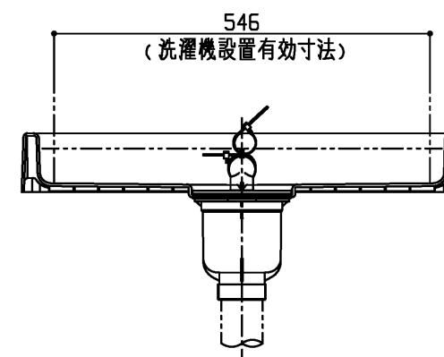
断面B-B
