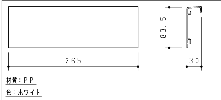
カバー (配管)
