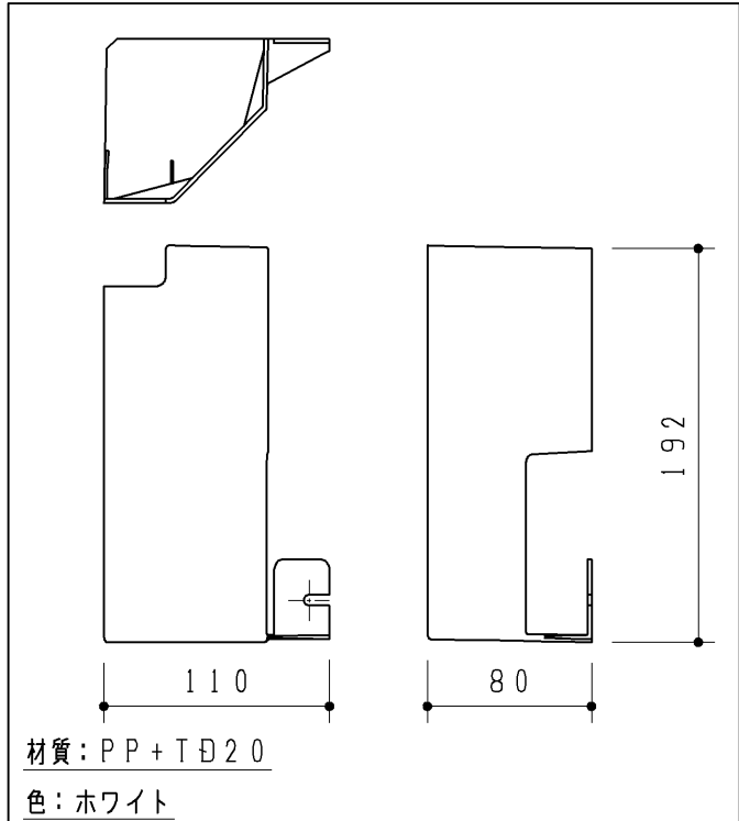
カバー (配管)
