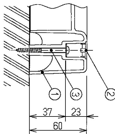
固定部詳細
