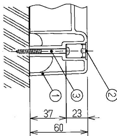
固定部詳細
