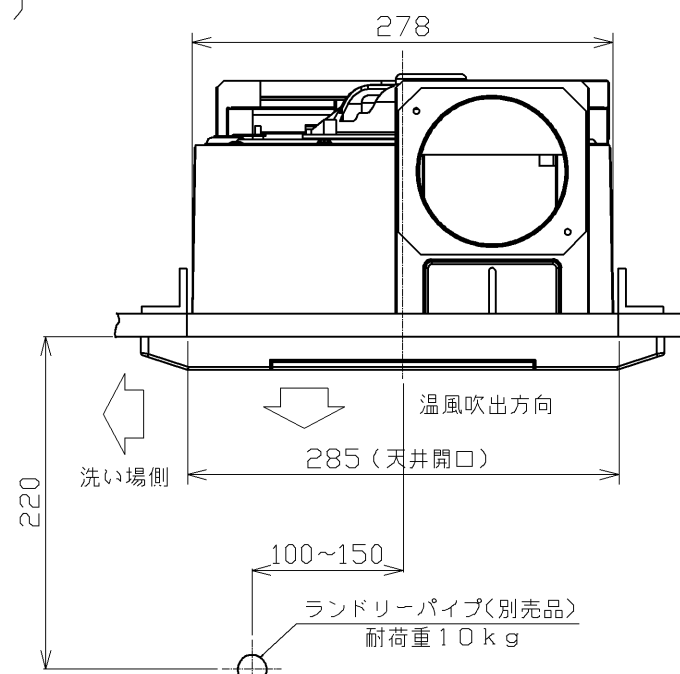
天井取付図 (1:5)
