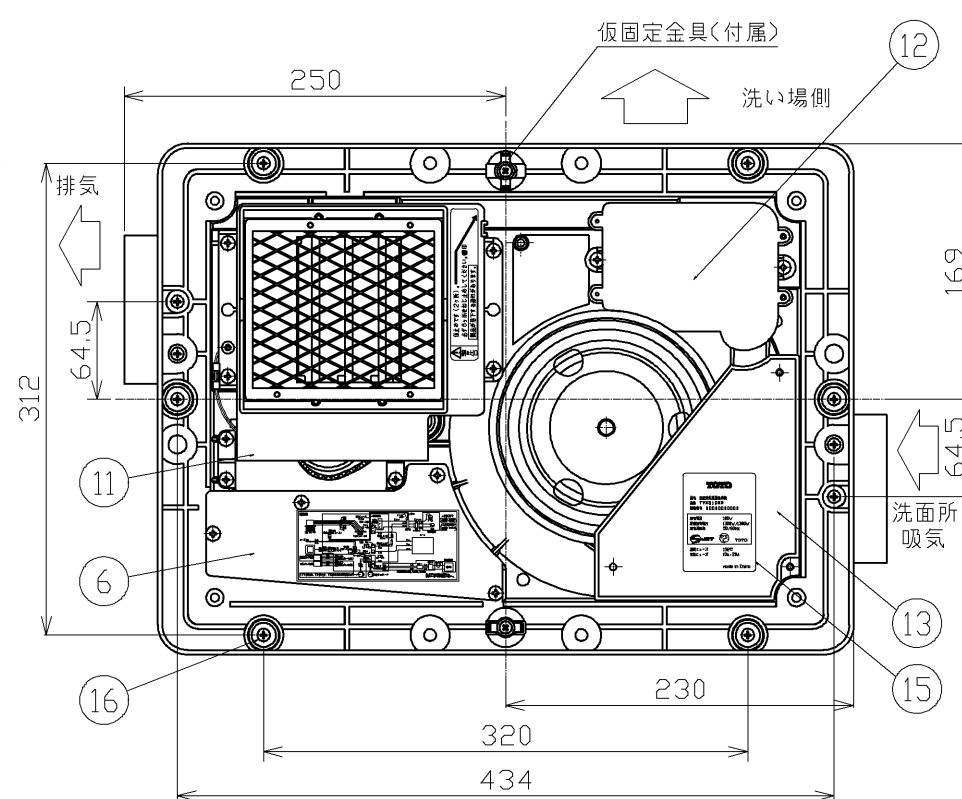
天井取付図 (1:5)
