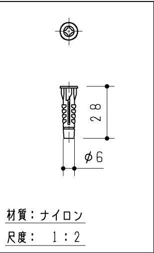
ボードアンカー 7ヶ
