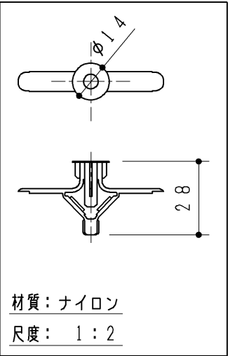
ボードアンカー 8ヶ
