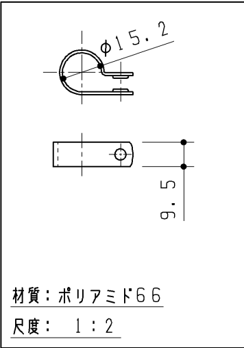
ホースクランプ 2ヶ
