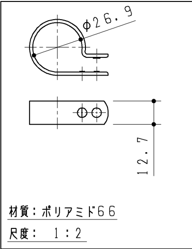
ホースクランプ 1ヶ
