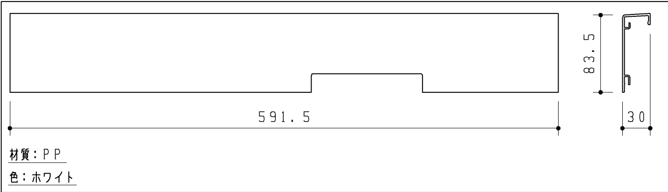
カバ- (配管)
