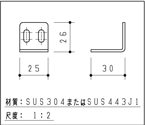
アングル 2ヶ
