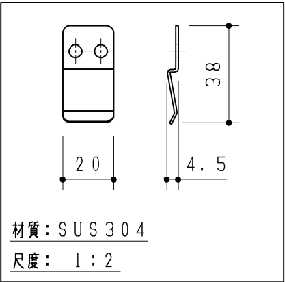
取付材 1ヶ
