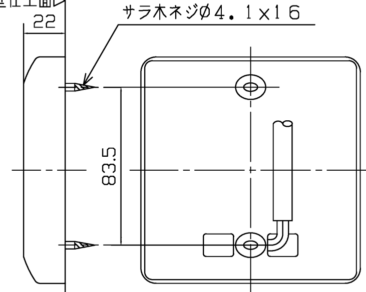
リモコン外観
