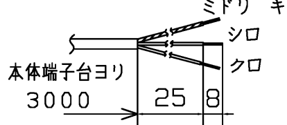
電源コード先端詳細
