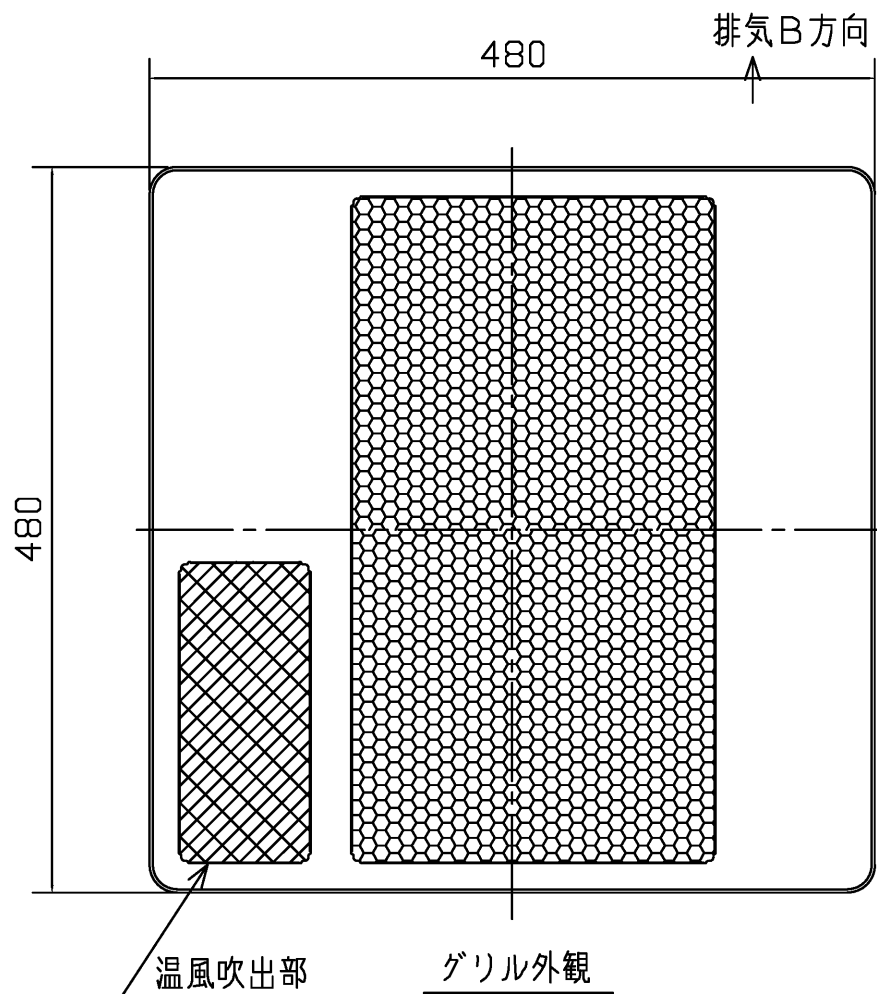
天井取付図
