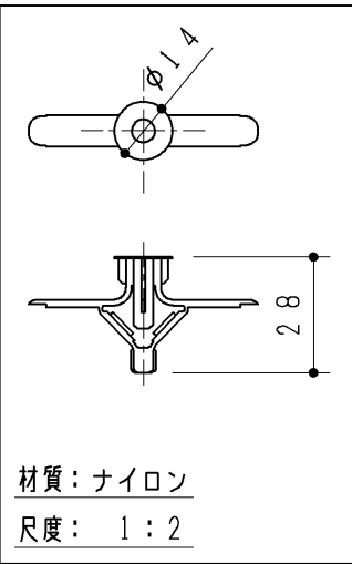
ボードアンカー 8ヶ
