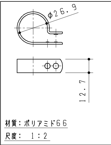
ホースクランプ 1ヶ
