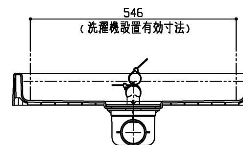
断面B-B
