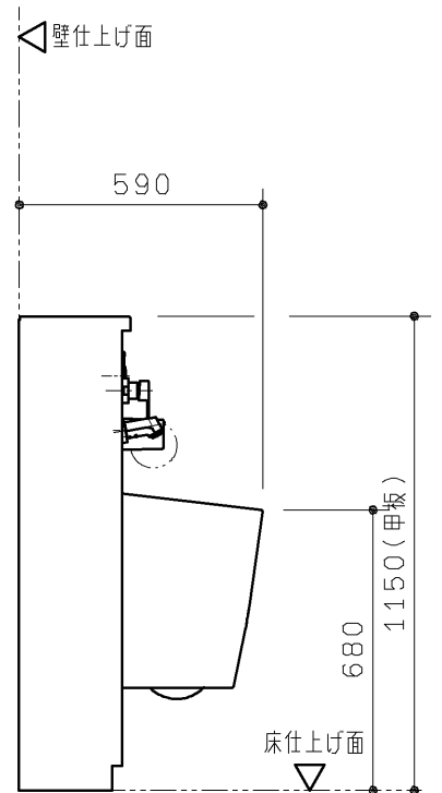
B矢視図
