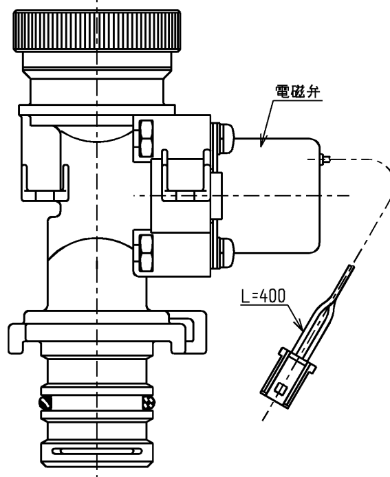
駆動部
