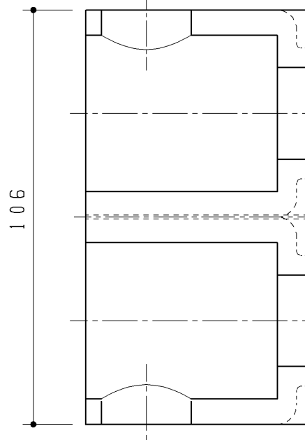
防露カバー（分岐金具部）
