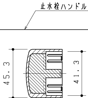
断面B-B
