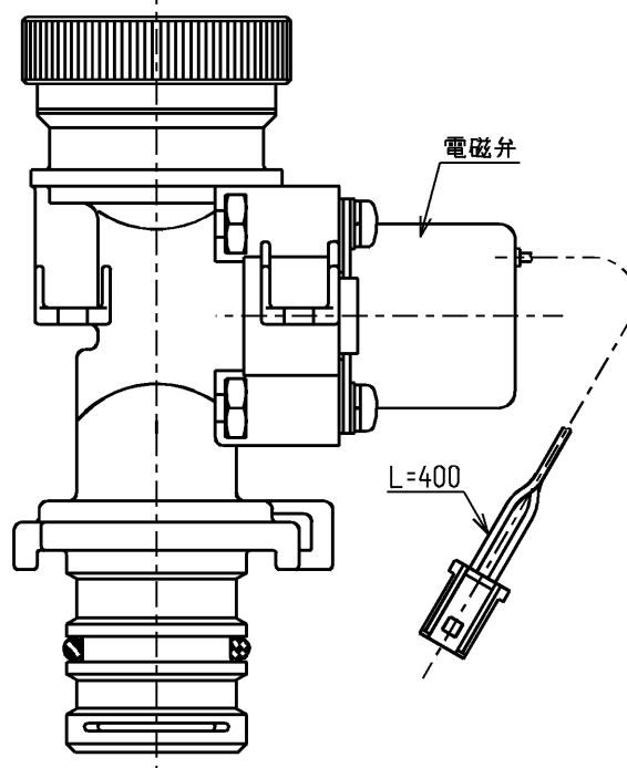
駆動部(2ヶ)
