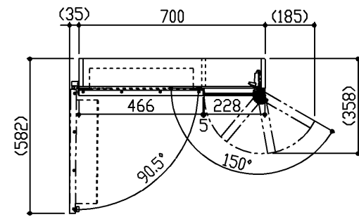
L0125R 軌跡図
