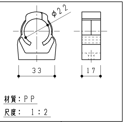
取付材 1ヶ
