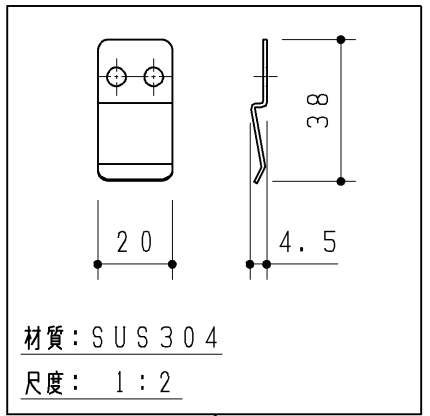
取付材 1ヶ
