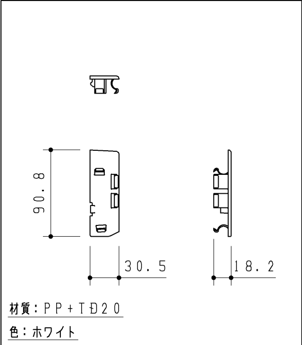
キャップ
