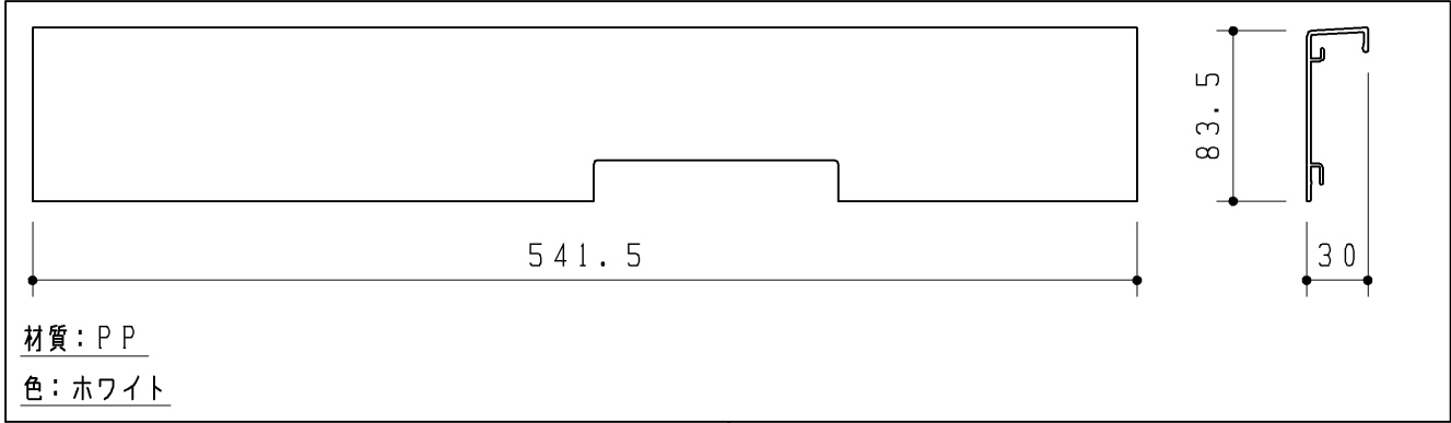
カバー（配管）
