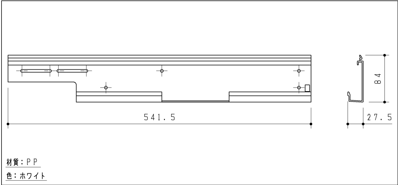
取付材
