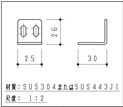
アングル 2ヶ
