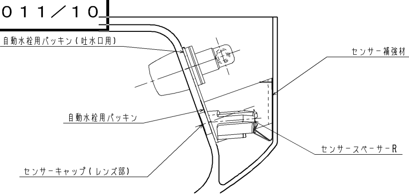
A部断面詳細図 (S=1:2)
