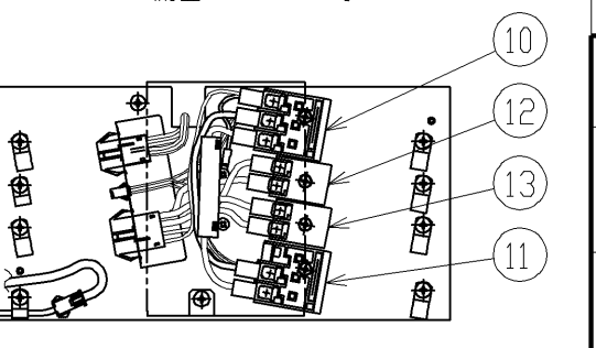
端子台配置図 ※端子台は換気ユニットの点検口側の側面にあります。
