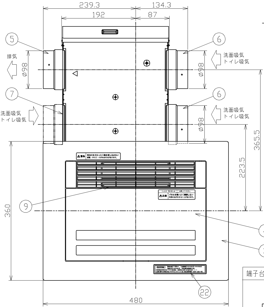
天井取付図 (1:5)
