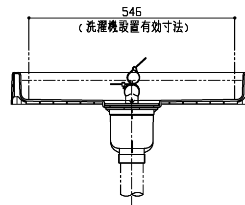
断面B-B
