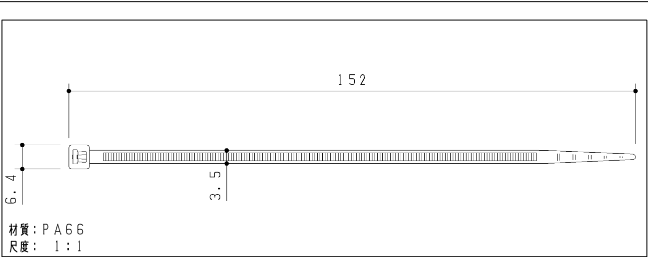
インシュロック (2ヶ)
