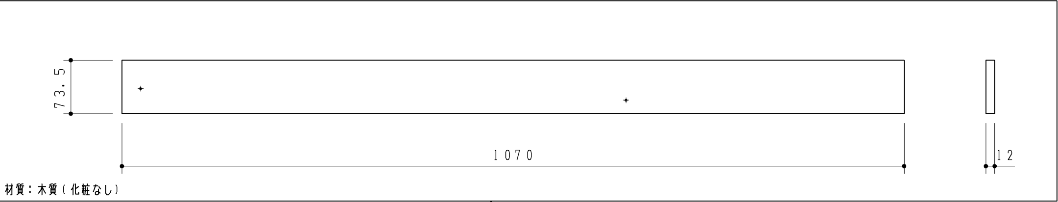
下段補強鉄
