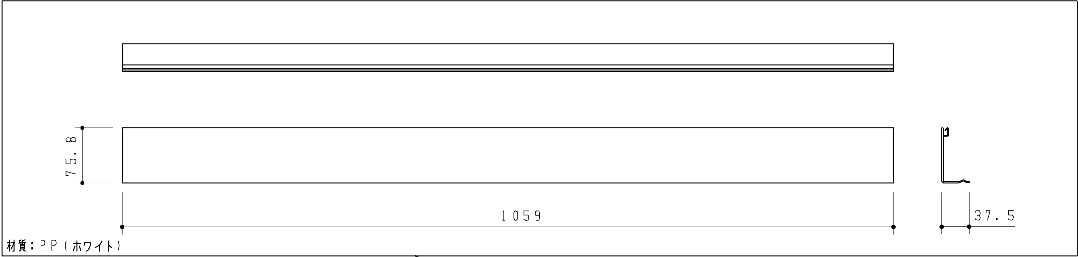
配管カバー
