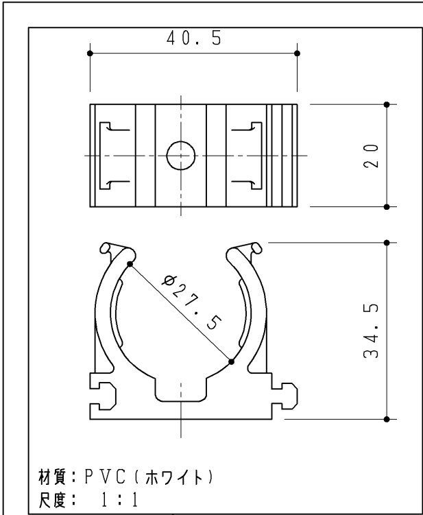
配管支持材 (2ヶ)
