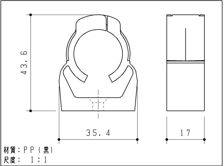
配管固定材 (3ヶ)
