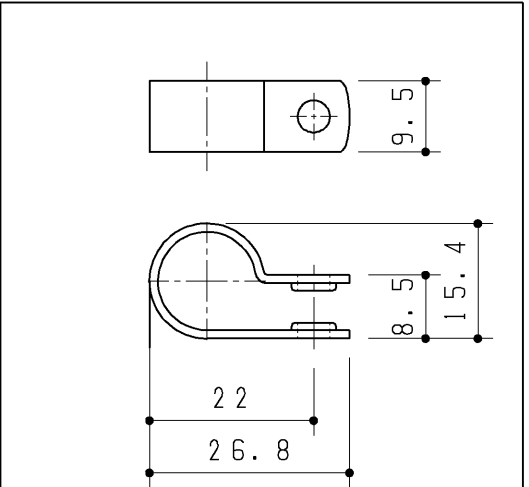
ホースクランプ (3ヶ)
