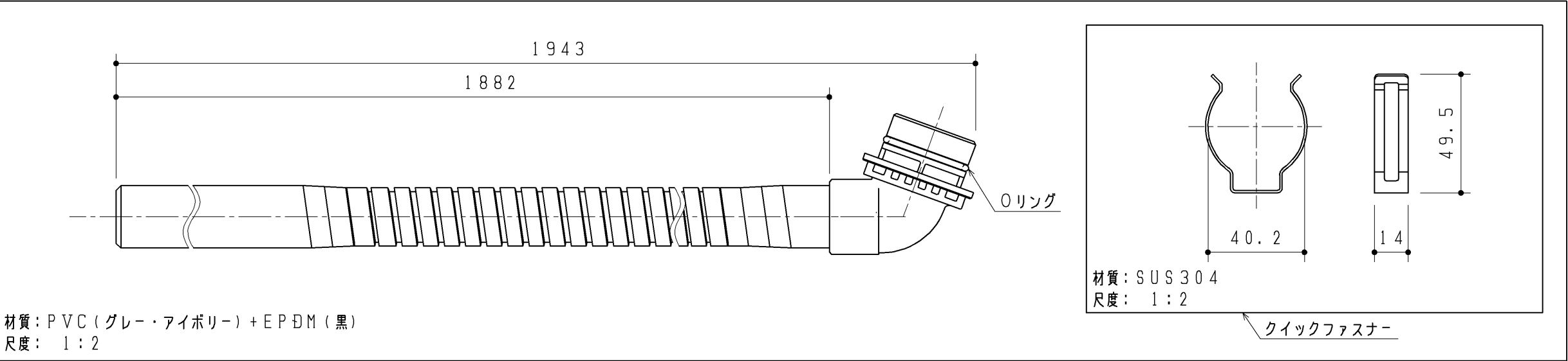
手洗排水ホースセット
