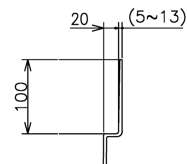
壁のせ部(防水リム部) 詳細
