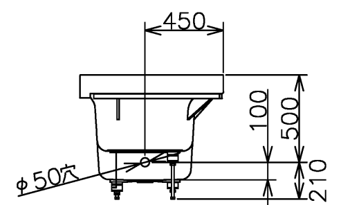
追焚穴あけ位置 ※ステップ下中央
