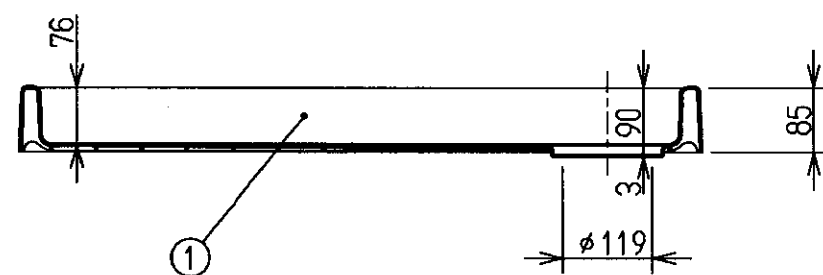
断面A-A
