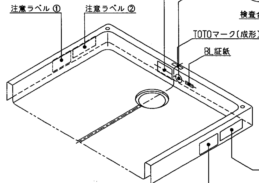
ラベル張付位置図
