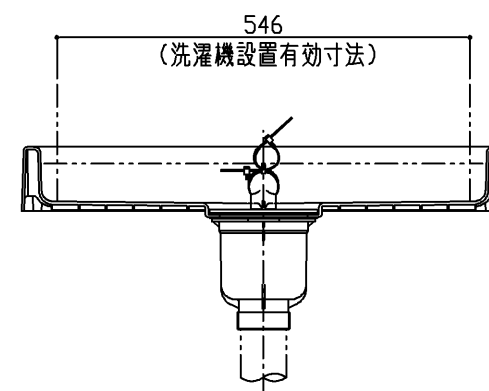
断面B-B
