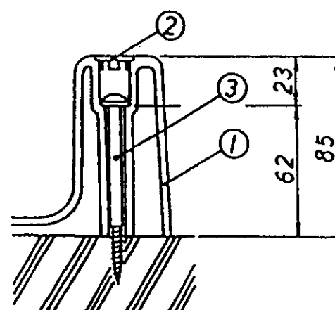
固定部詳細
