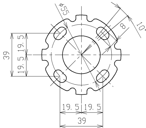
取付座詳細図( 1: 2 )
