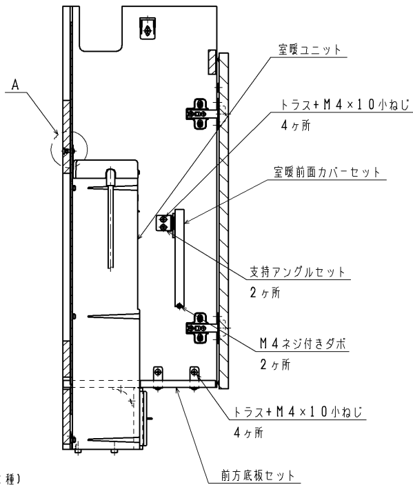
室温ユニット固定詳細
