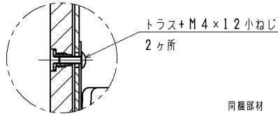
A部詳細 (S=1:2)
