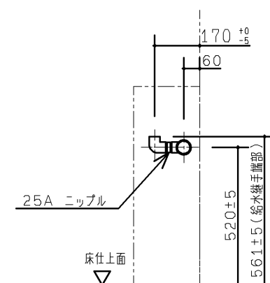
Q 视图
