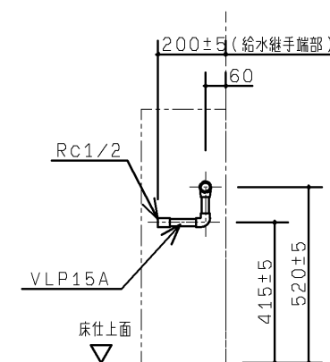
R 視図
