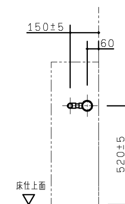
P 視図
