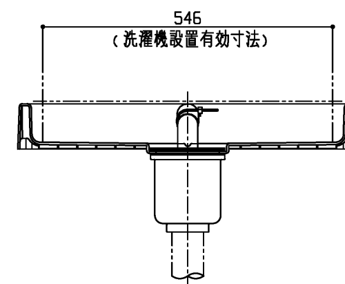
断面B-B
