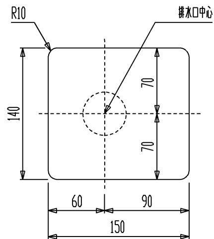
カウンター切込寸法
