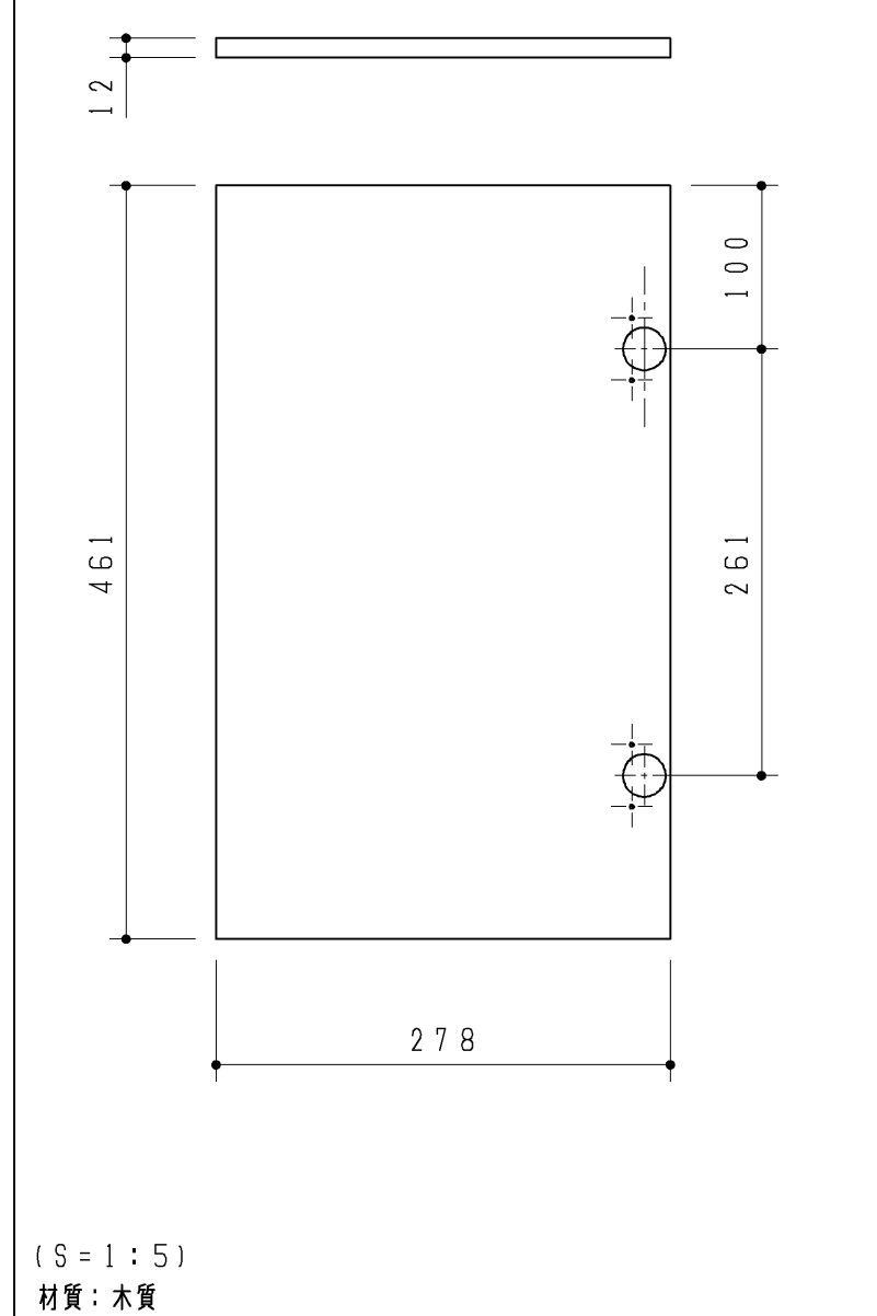
丁番用スペーサー (2ヶ)
