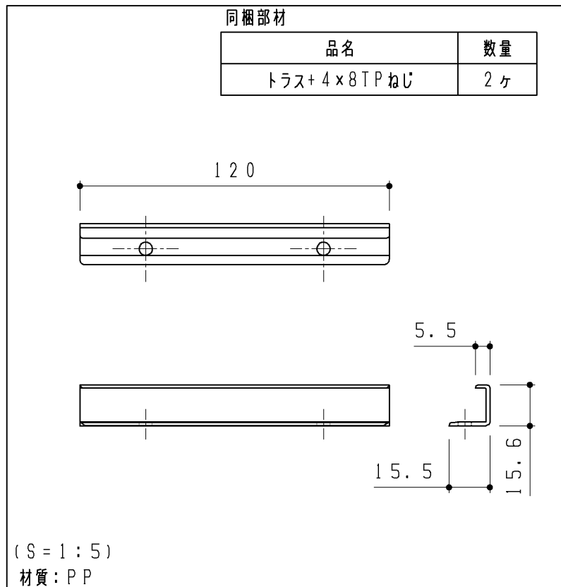
キャップセット
