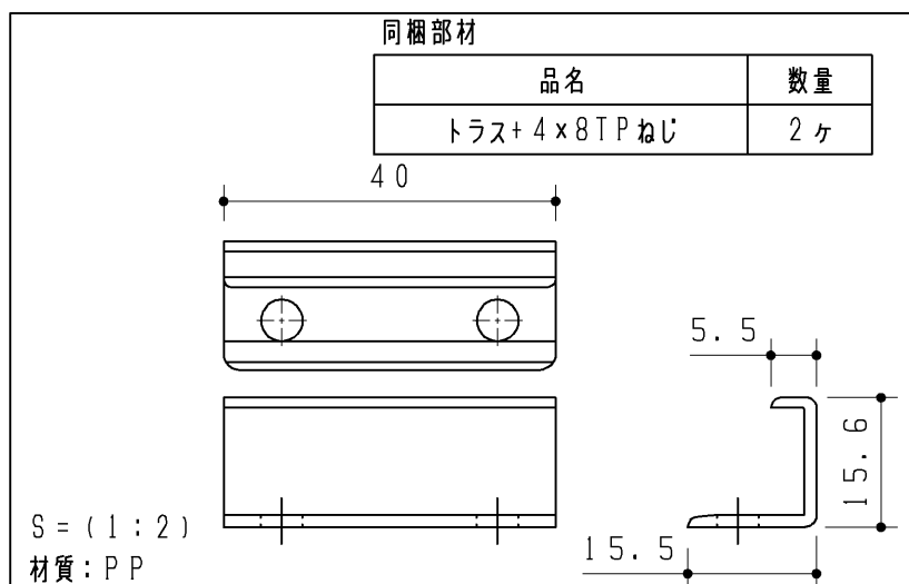
キャップセット
