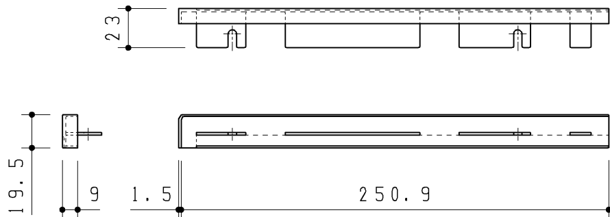
天板キャップセットL
