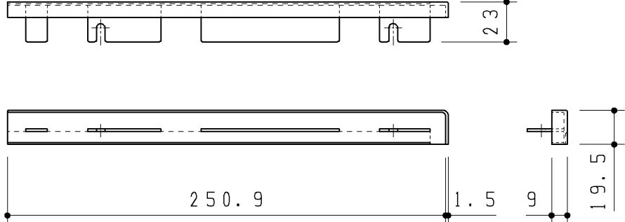
天板キャップセットR
