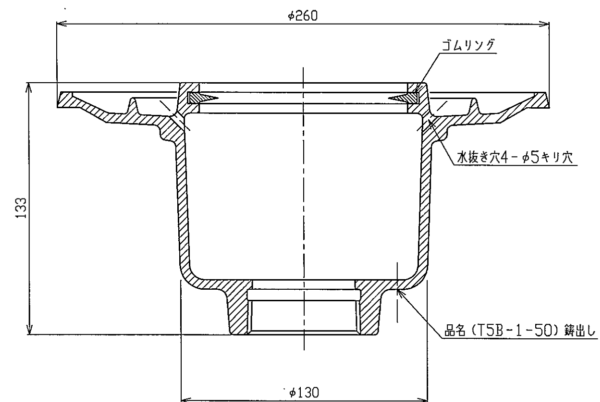
A-A断面図
