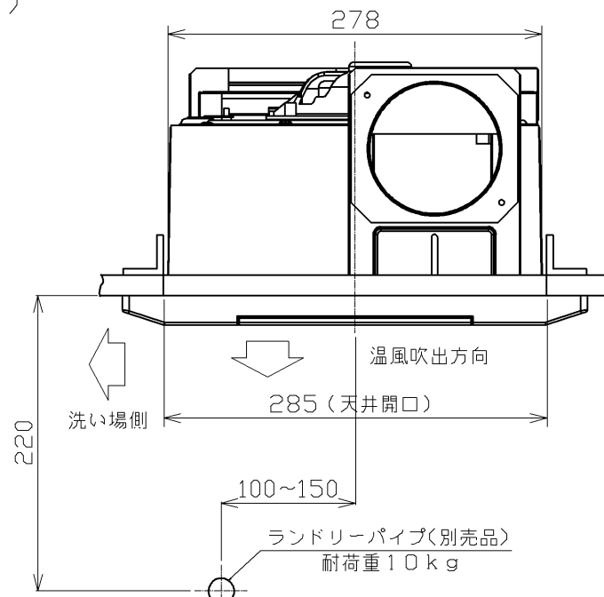
天井取付図 (1:5)
