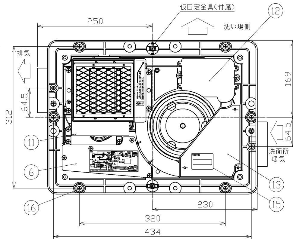
天井取付図 (1:5)
