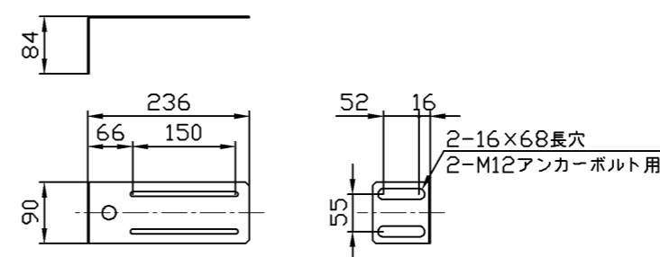
■壁固定金具 (付属品) (1:10)
