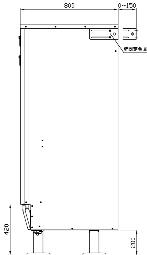
■壁固定金具 (付属品) (1:10)
