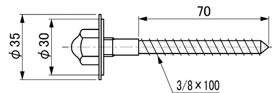
取付ボルト×2セット付(尺度1:2)
