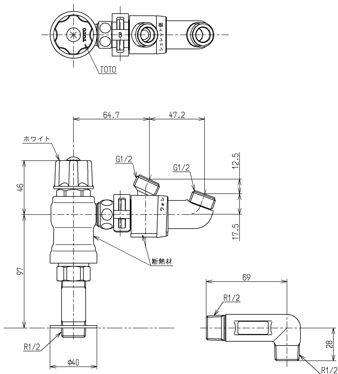
壁給水用エルボ
