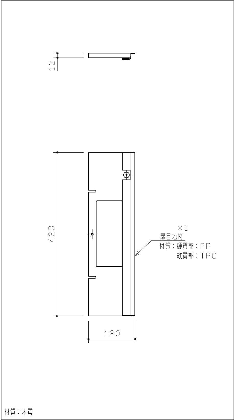
裏扉セット
