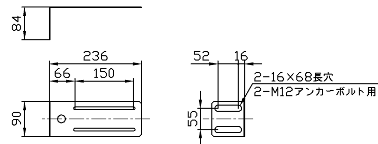
■壁固定金具（付属品）（1:10）
