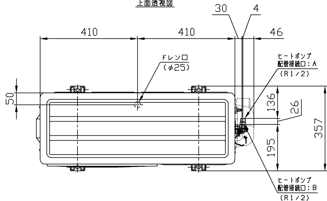
配管取出位置 上面透視図
