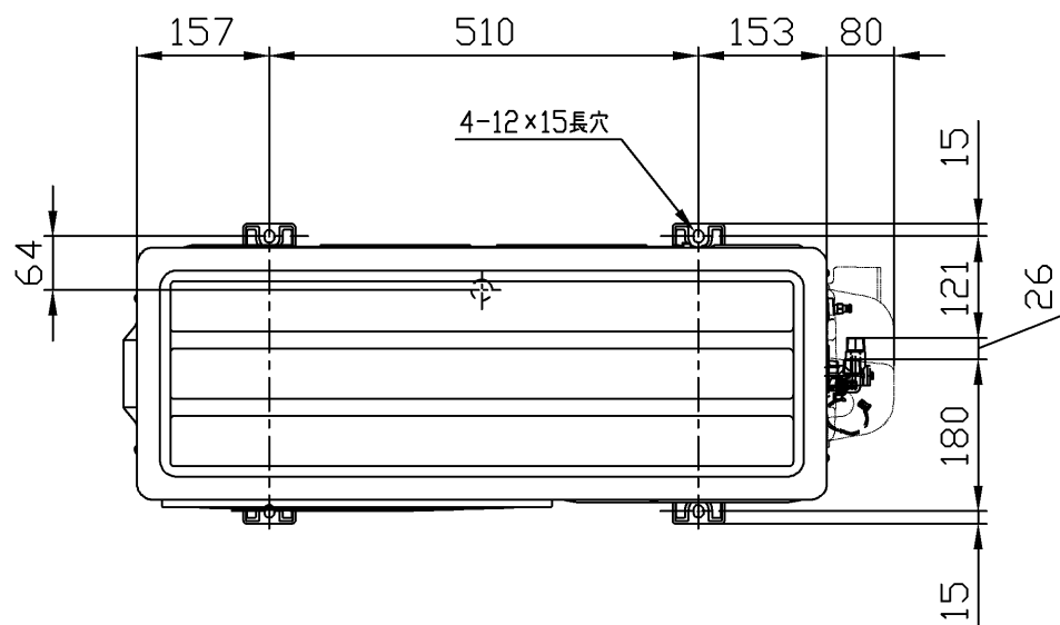
基礎ボルト位置 上面透視図
