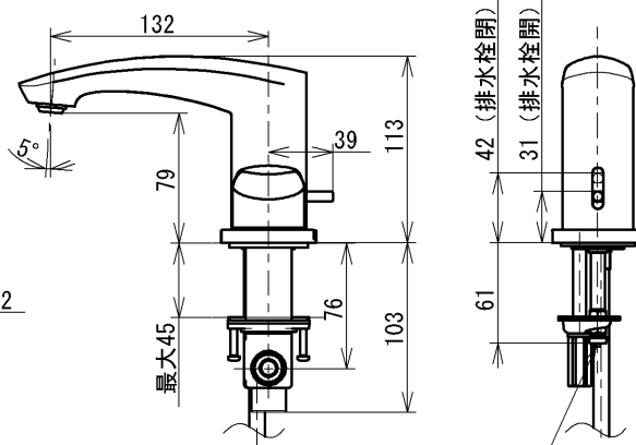
排水金具接続部 (専用のワンプッシュ式 排水金具とセットしてください。)
