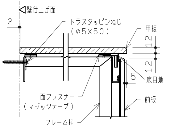
甲板部納まり詳細図（S＝1：5）
