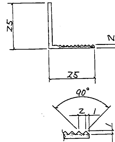
詳細図(3)
