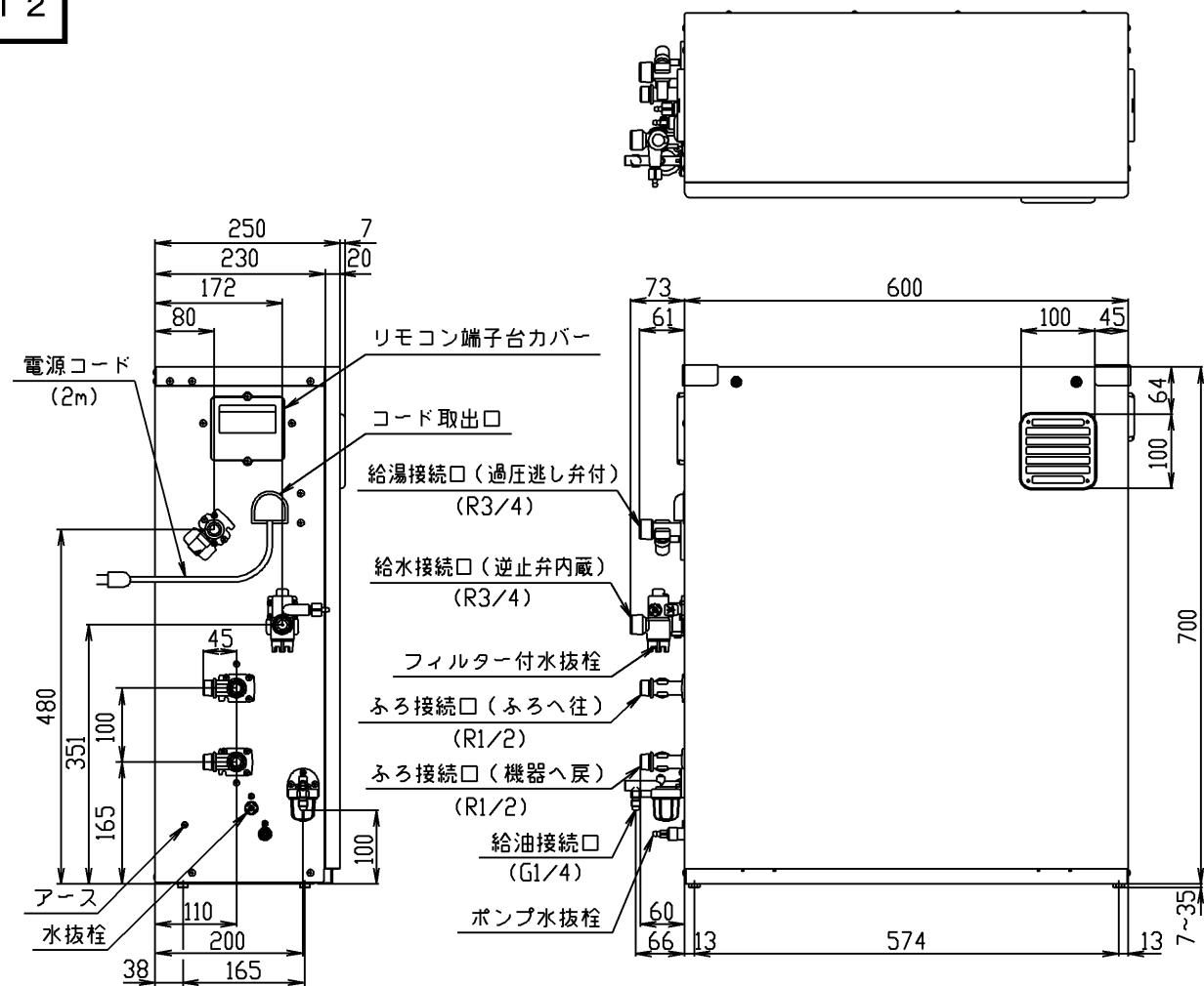
注 給水接続口に逆止弁内蔵
