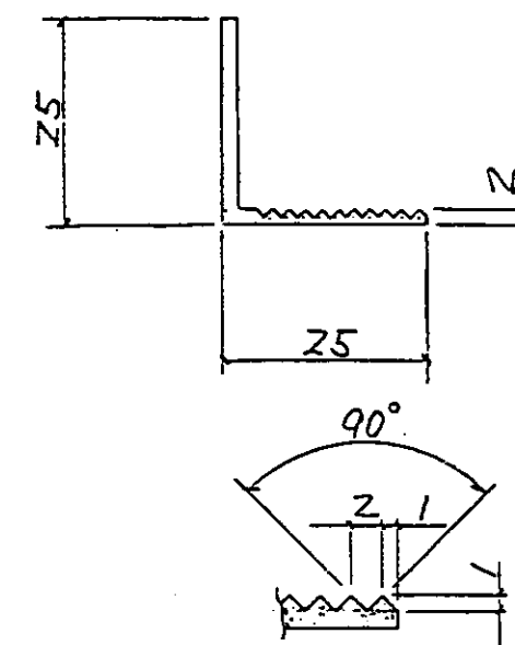
詳細図(3/1)
