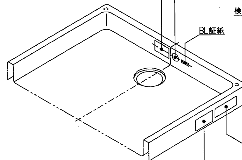
ラベル張付位置図
