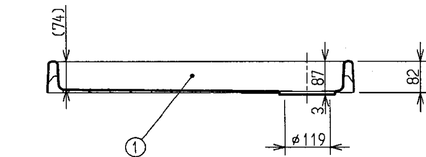
断面A-A
