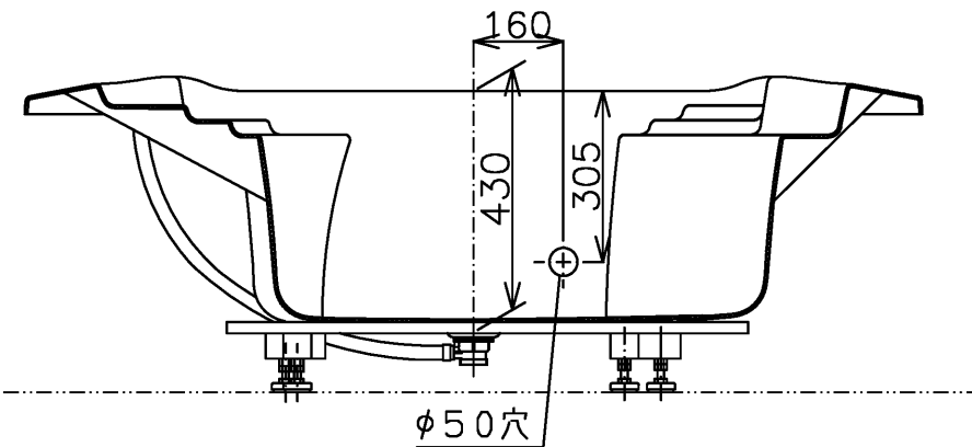
断面A-A
